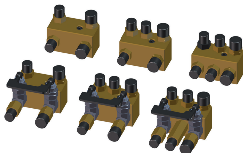
UCW-0475-59-00-00-0 Регулируем държач за машинна горелка φ 30mm (1.18")
